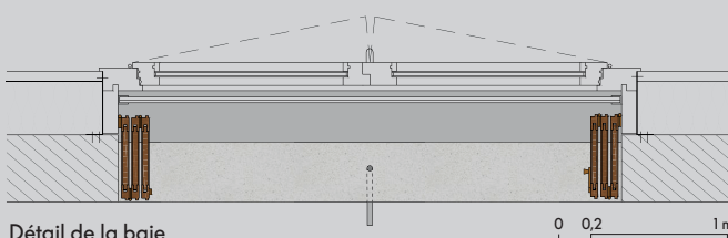
Détail de la baie
